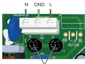
Selectores de regulación de la velocidad variable
