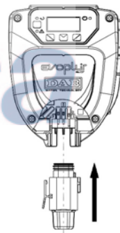
4 pav. Maitinimo jungties prijungimas.
