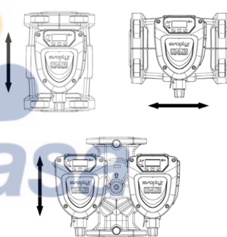
Abbildung 1: Montageposition
