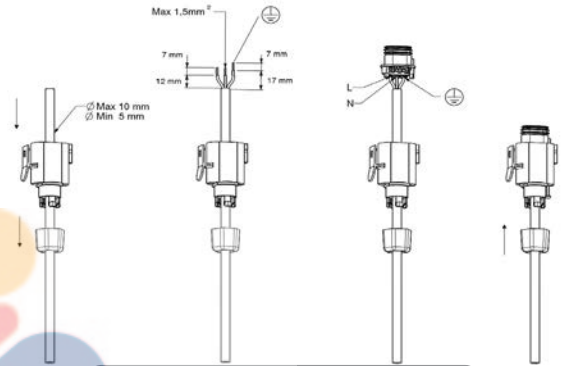
Resim 3: Güç besleme konektörüne kablo çekilmesi
