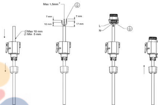
3.sz.ábra: elektromos csatlakozás kábelzése
