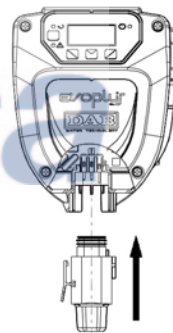
Afbeelding 4: Aansluiting voedingsstekker
