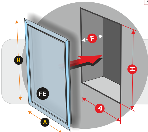
DIMENSIONES DEL HUECO PARA INSTALACIÓN EMPOTRAMIENTO
